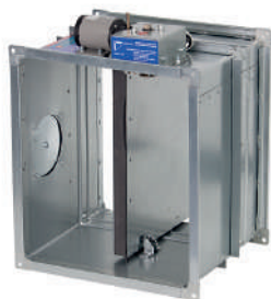
КЛОП-2(60) с электромагнитным приводом и тепловым замком
